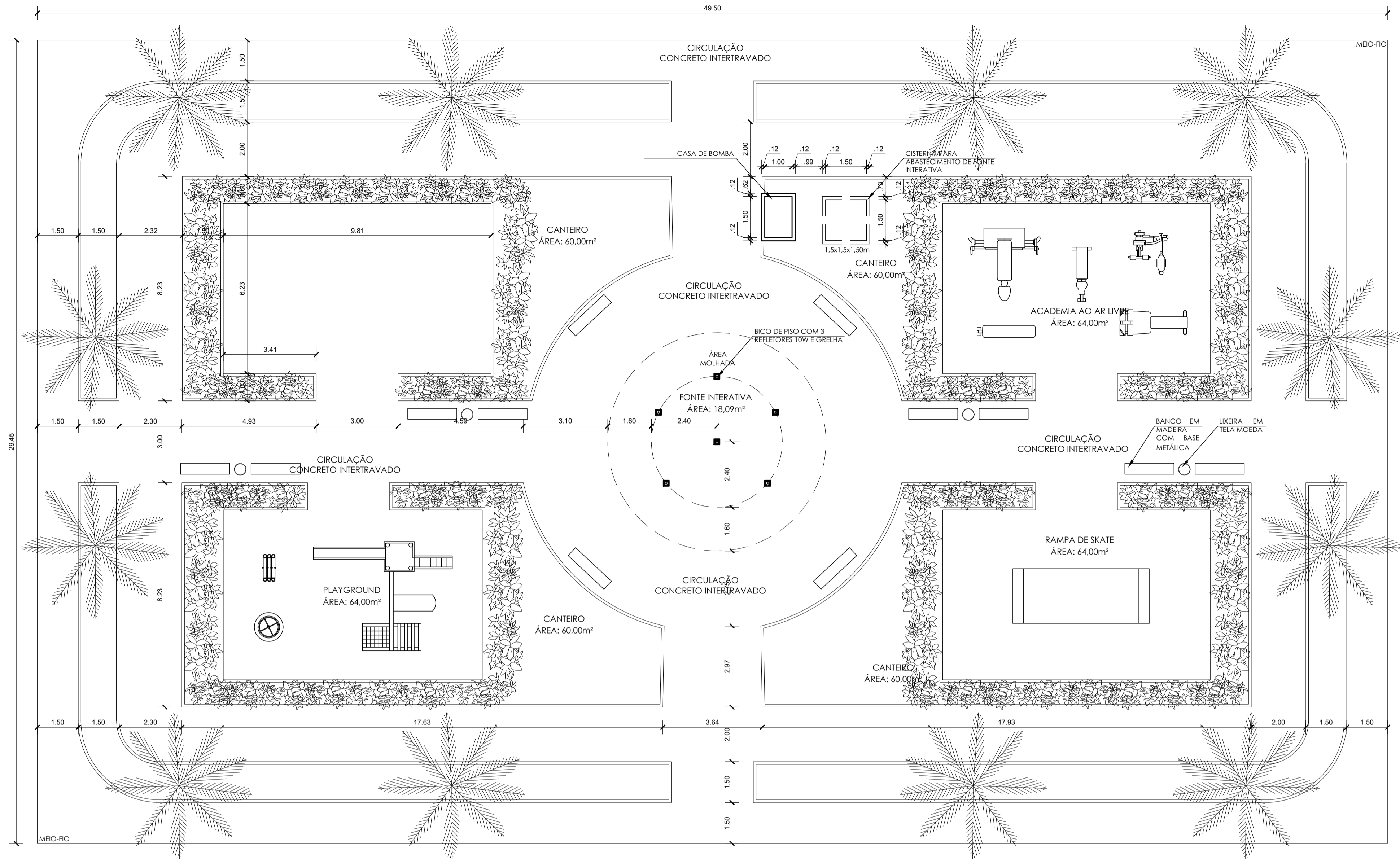
PLANTA BAIXA - PRAÇA SÃO PEDRO ESCALA 1:100
