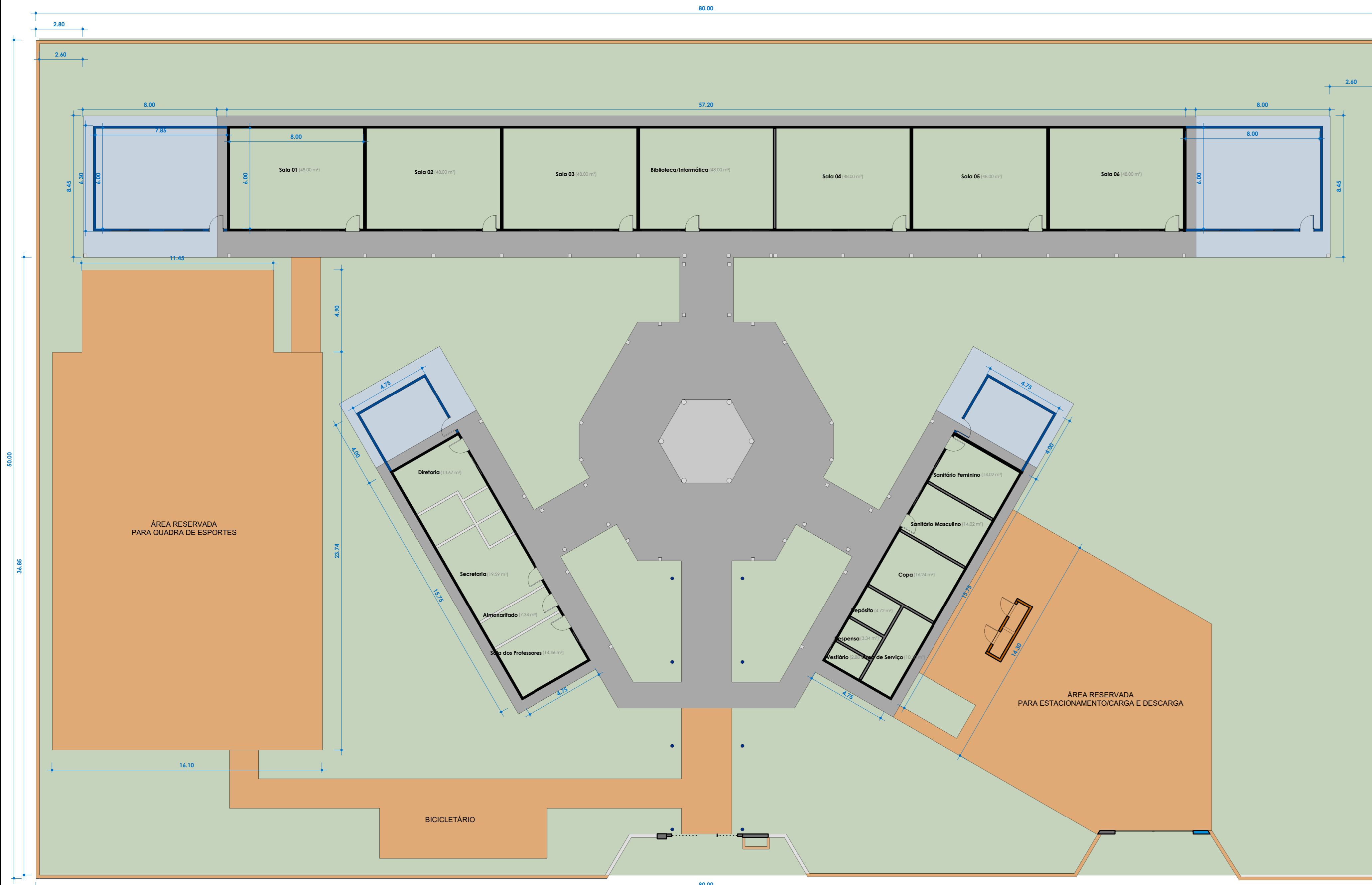
1 Planta de Piso 1:150
